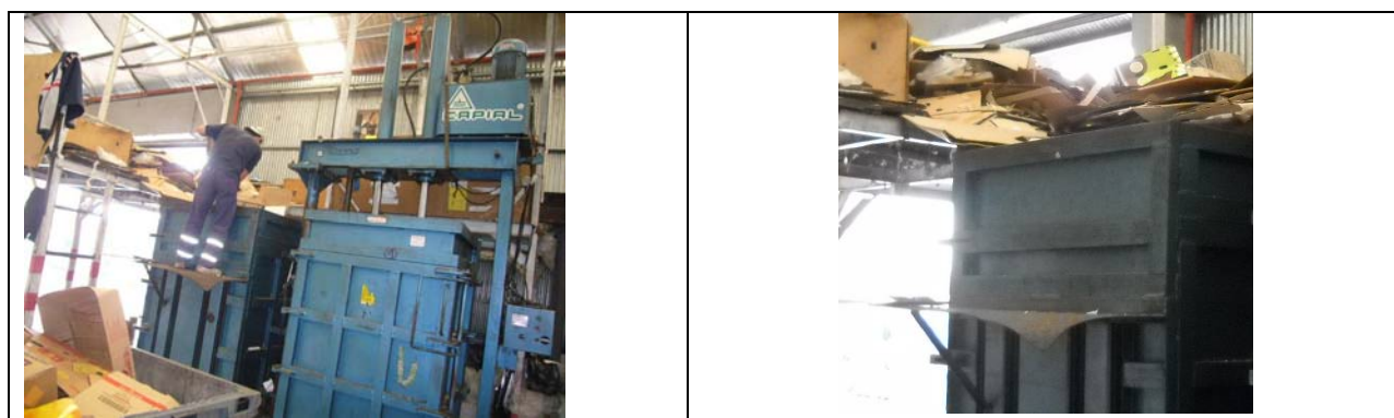
Fotos N° 20 y 21: Enfardadora doble cajón y detalle de plataformas metálicas agregadas de tipo precario.
